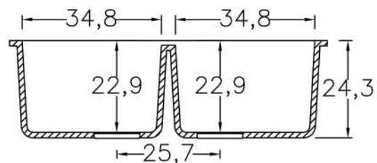
Corte Lateral
