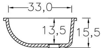
Corte Lateral
