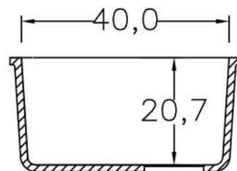
Corte Lateral
