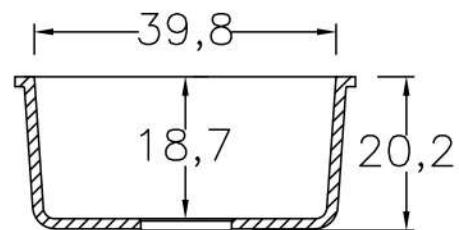
Corte Lateral
