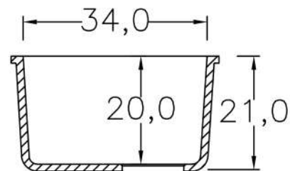
Corte Lateral
